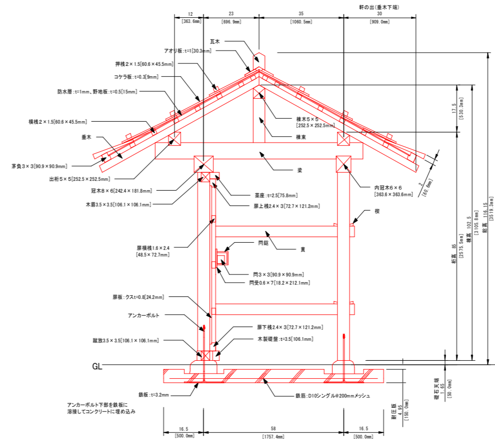
門断面図
