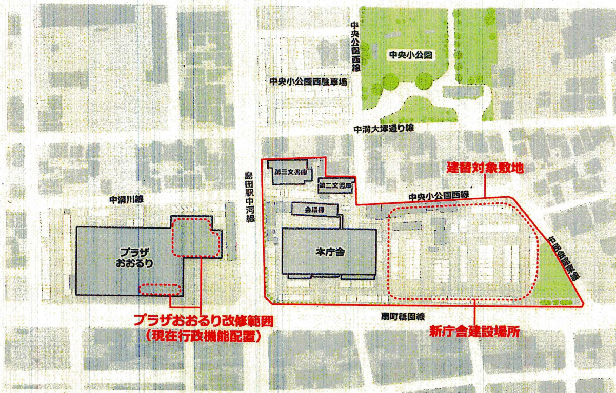
現況配置図
