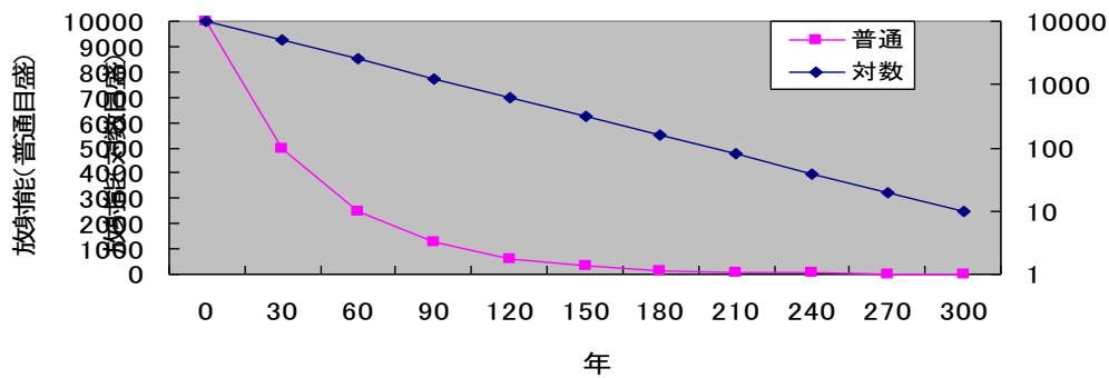
図5 半減期30年の例
