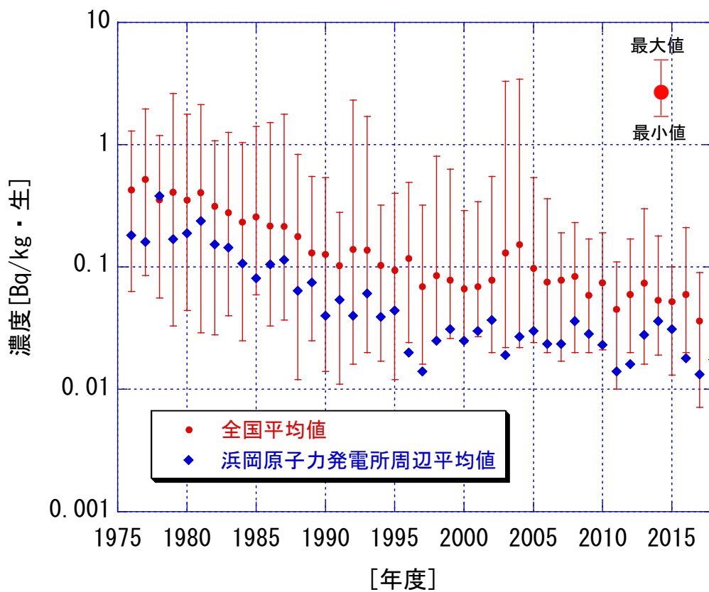
図8 大根中 Sr-90 濃度
