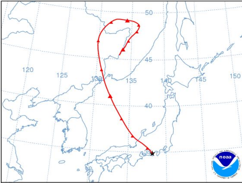
図6 後方流跡線解析
