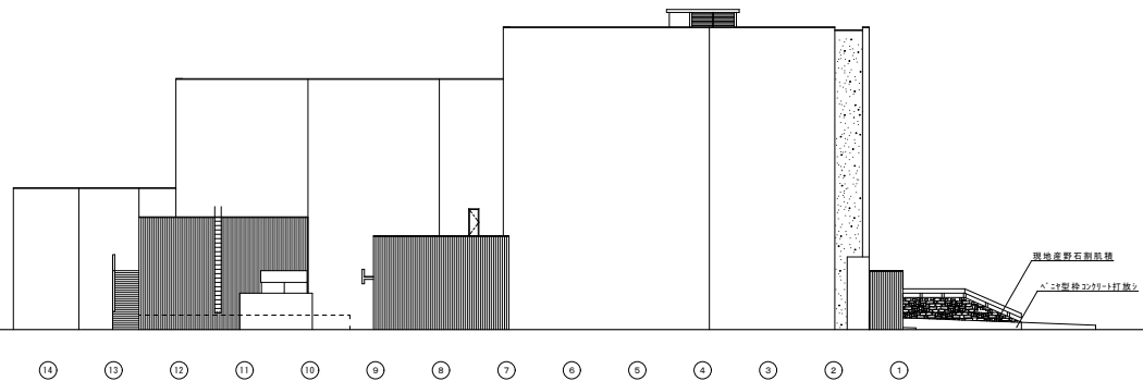
北面立面図 S = 1 / 200
