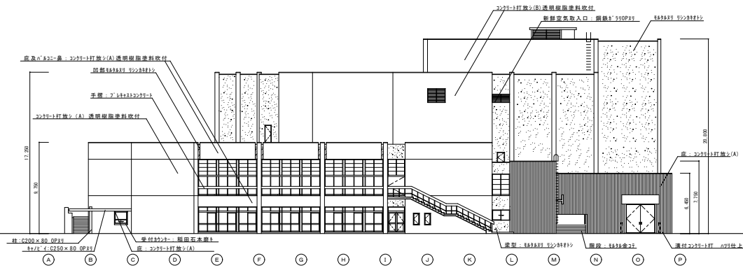
東面立面図 S = 1 / 200
