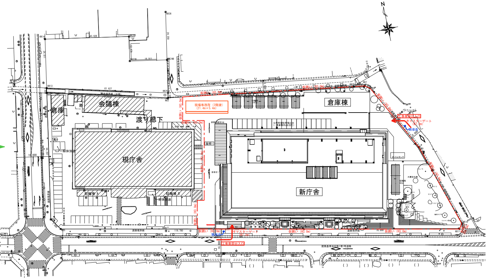
STEP2 : I 期工事 (新庁舎建設、新庁舎周辺外構整備)
