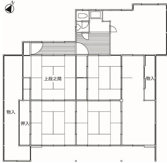
平面図
