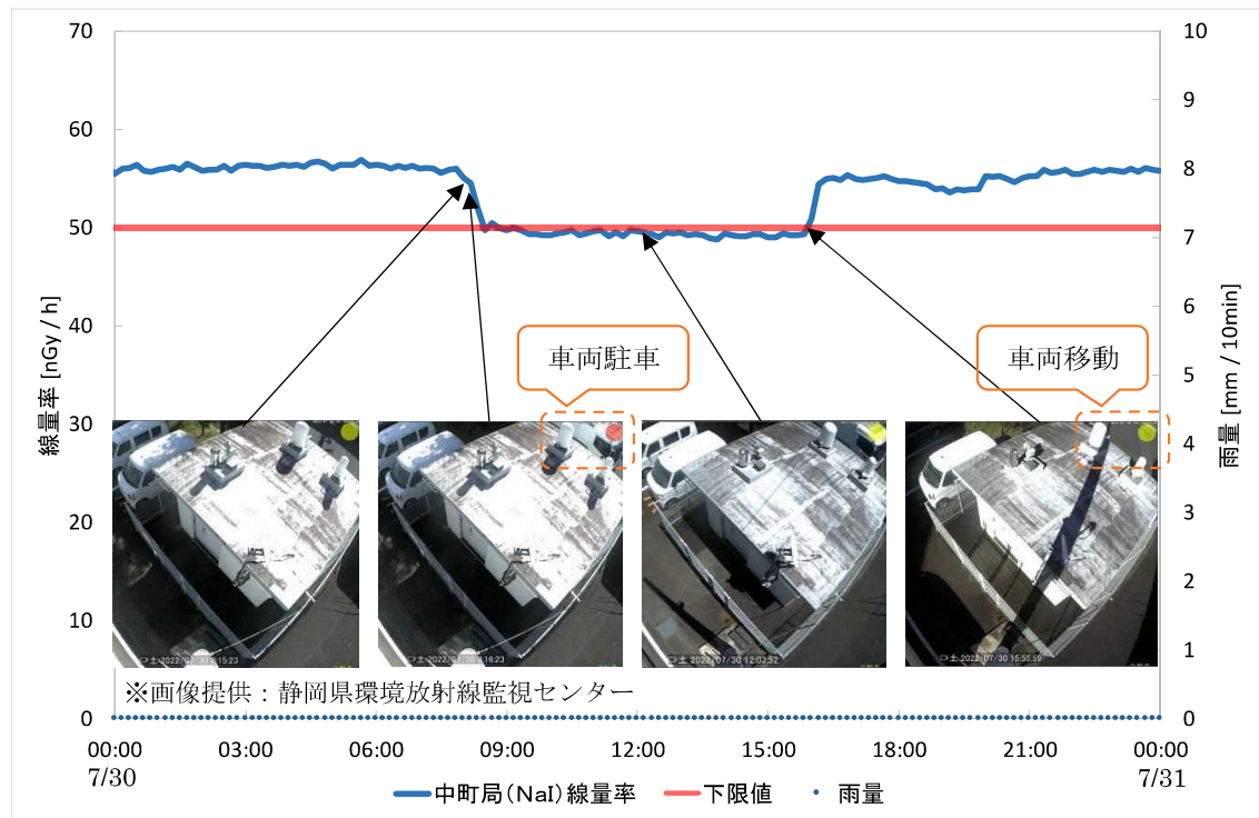
図 1 中町 MS の空間放射線量率時系列変化
