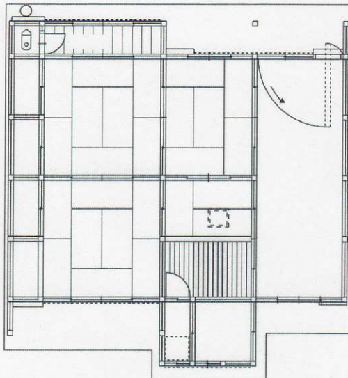
図20 仲間の宿平面及び立面図
