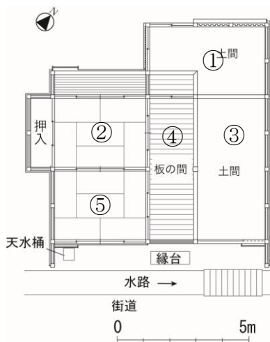
図 36 十番宿平面図
