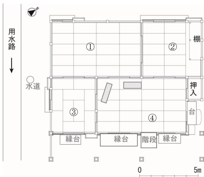
図 33 川会所平面図
