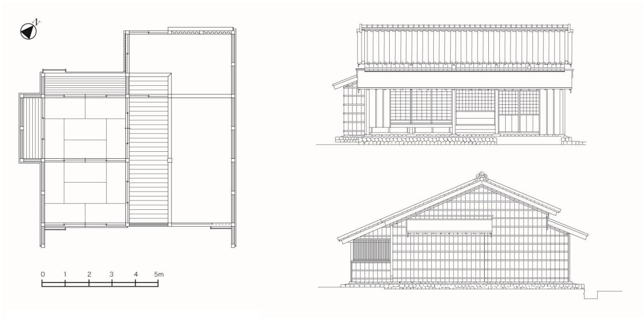
図 22 十番宿平面・立面図
