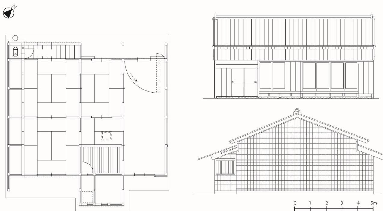
図20 仲間の宿平面・立面図
