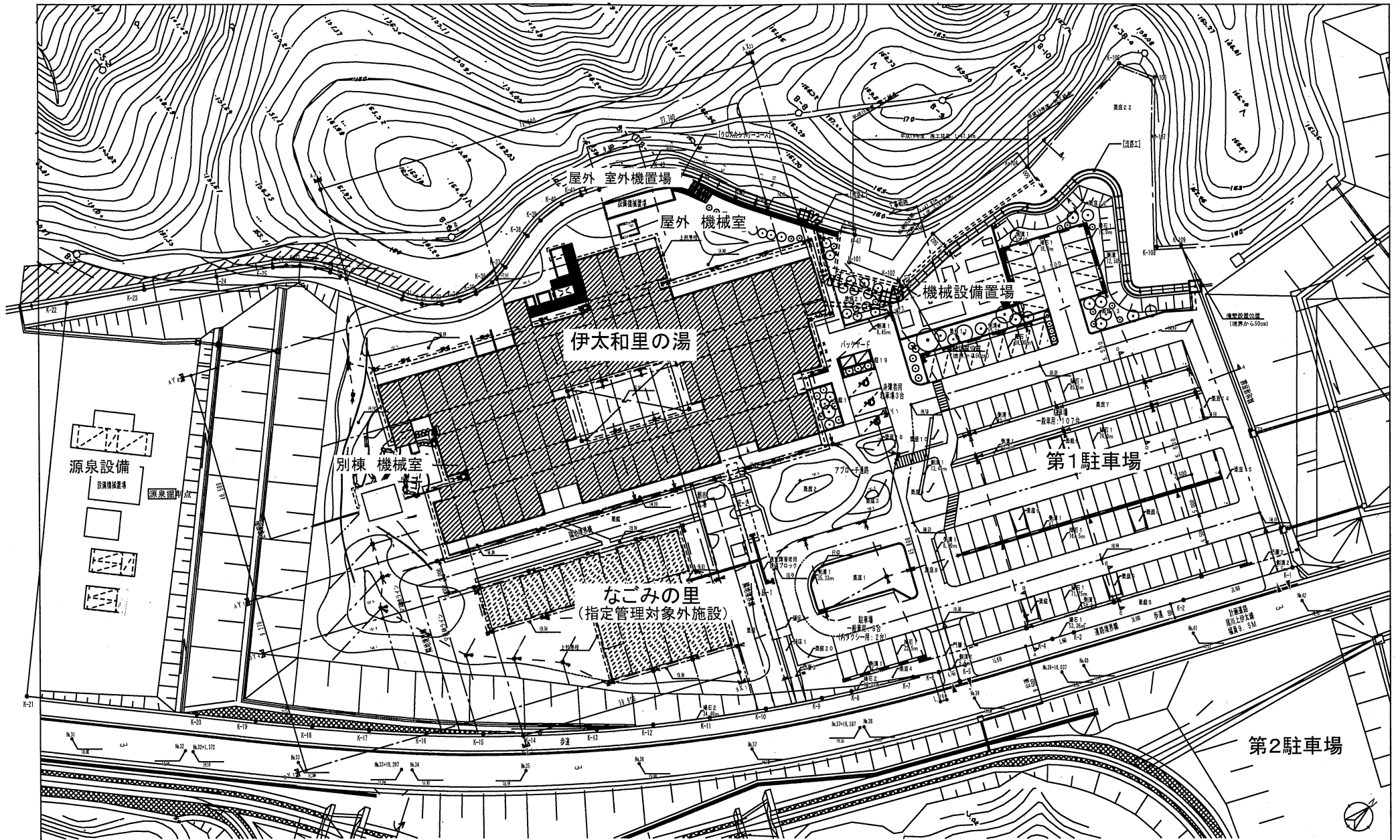
田代の郷温泉 伊太和里の湯 配置図
