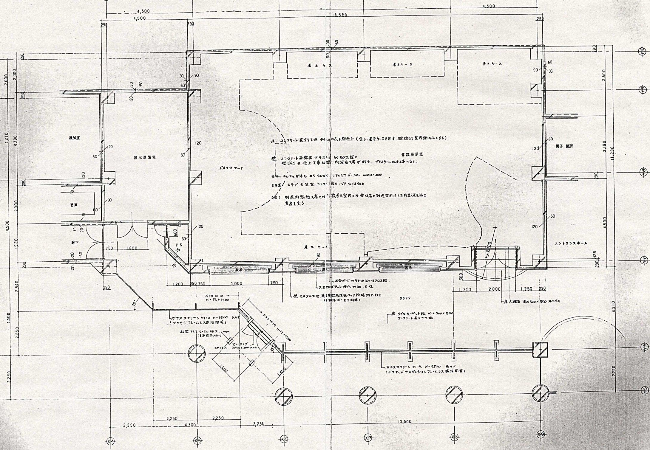
多設展示室 展示準備室 平面詳細図 S1/50
