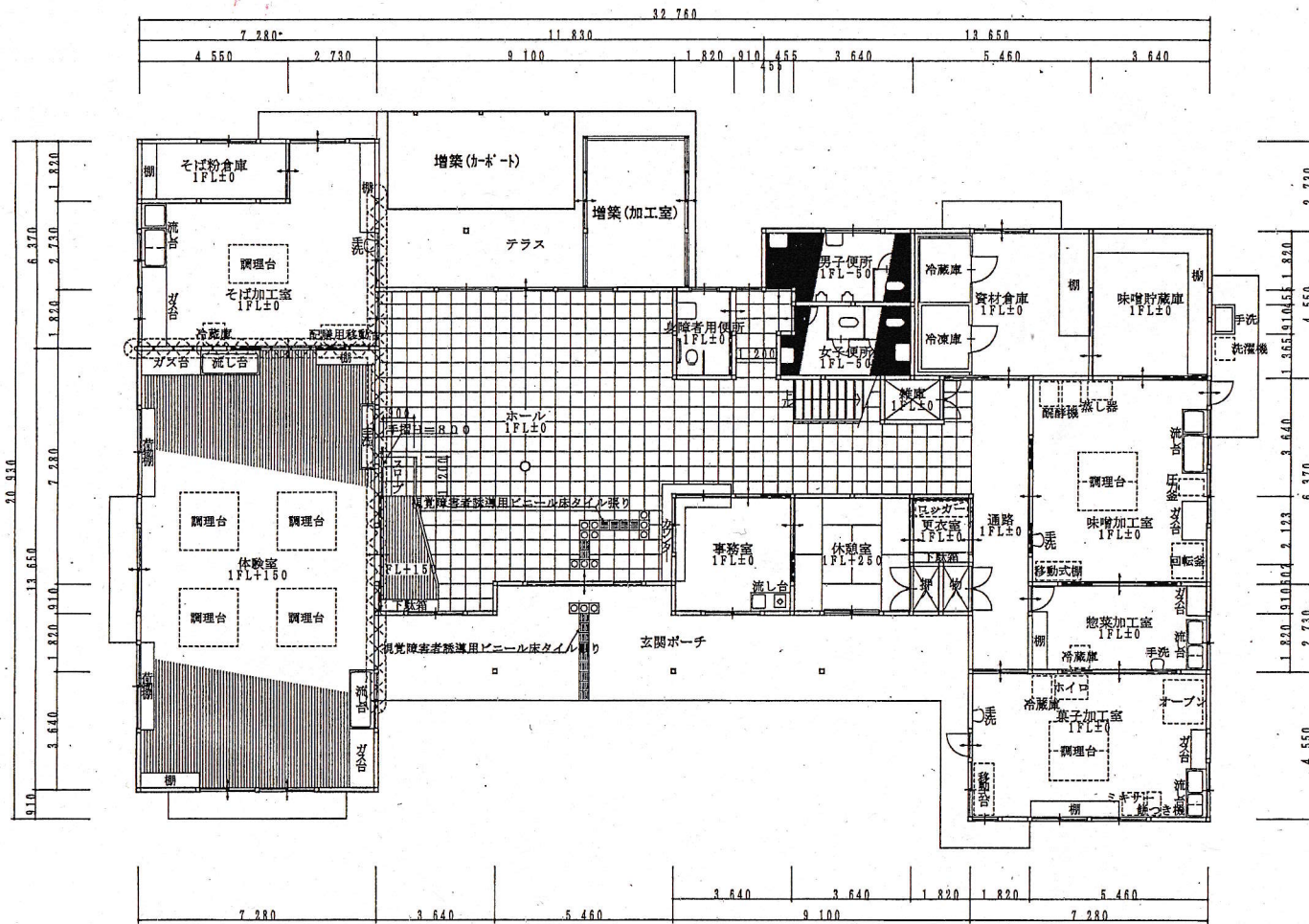
1階平面図 S=1:150
