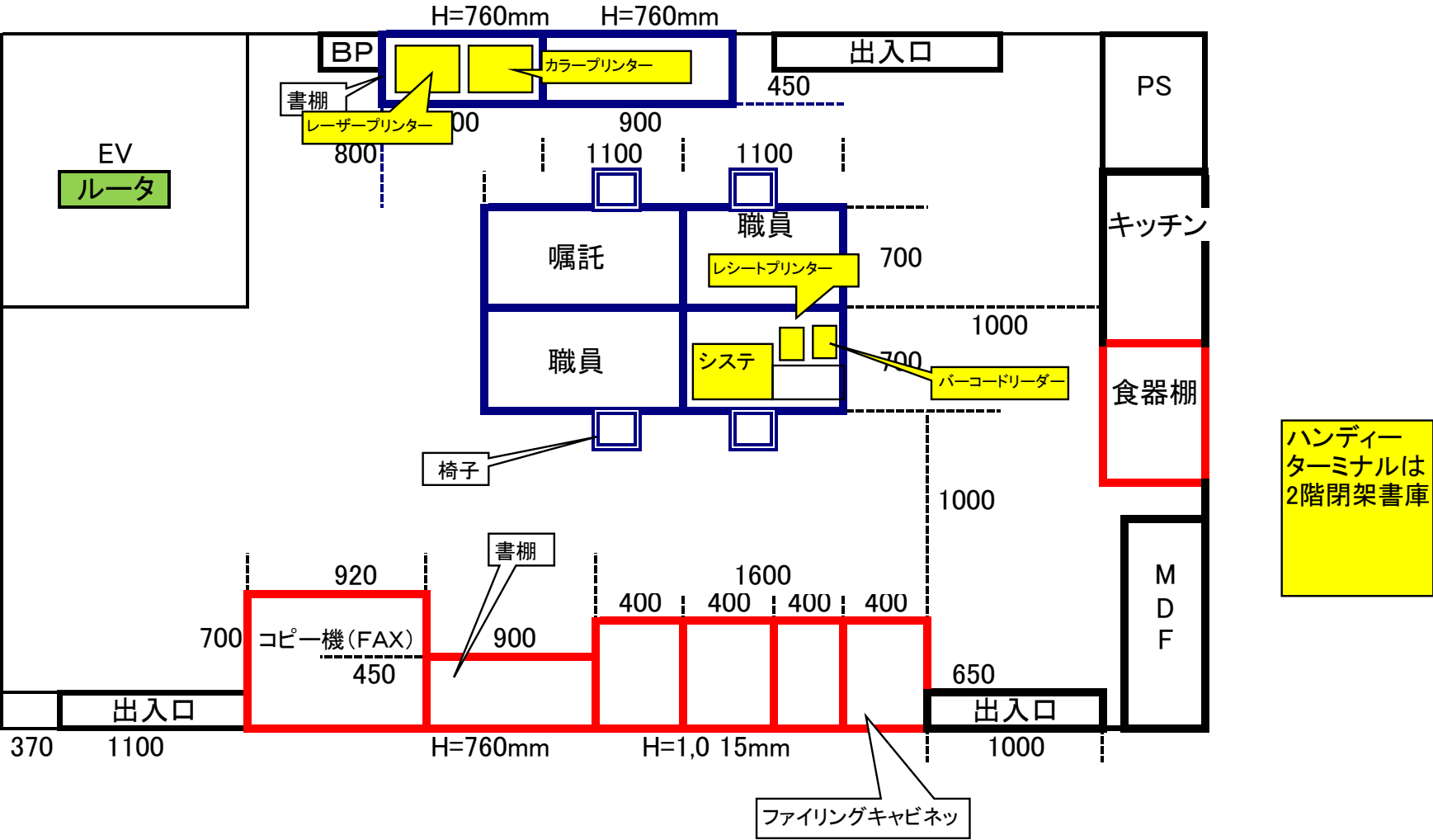
川根図書館事務室機器等配置図
