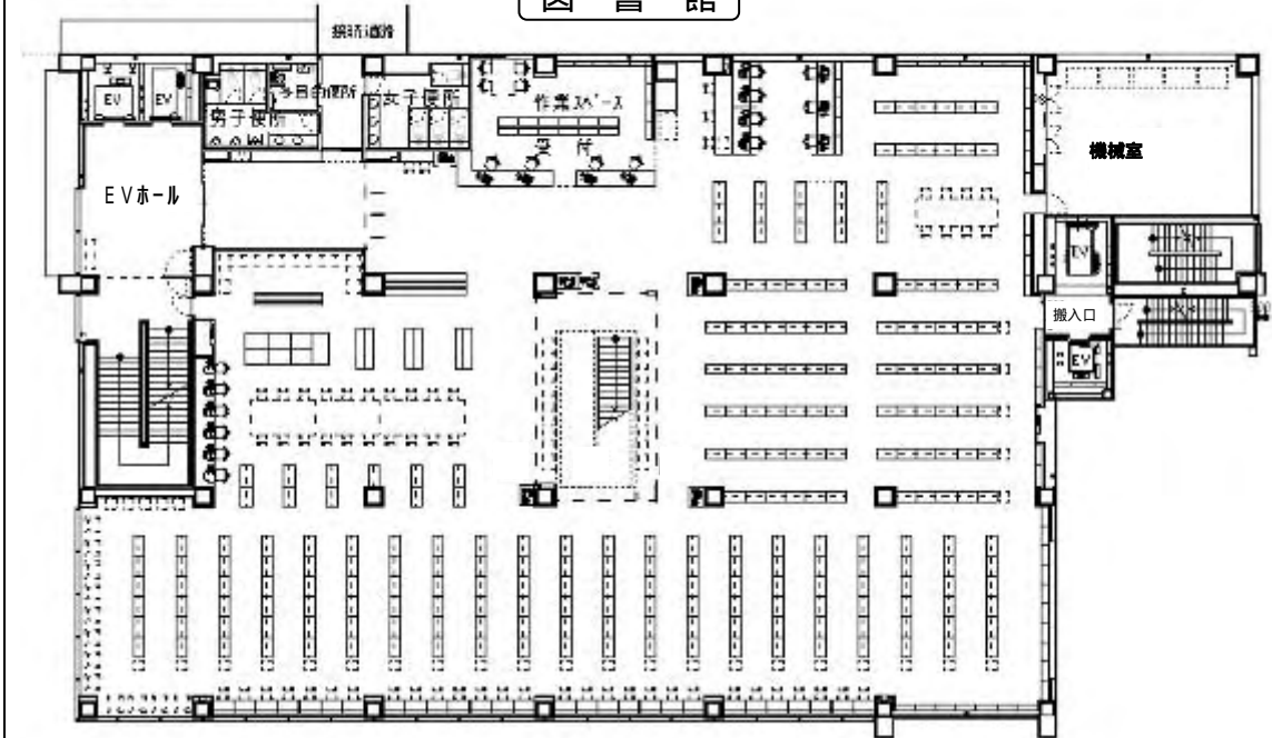
2階平面図
