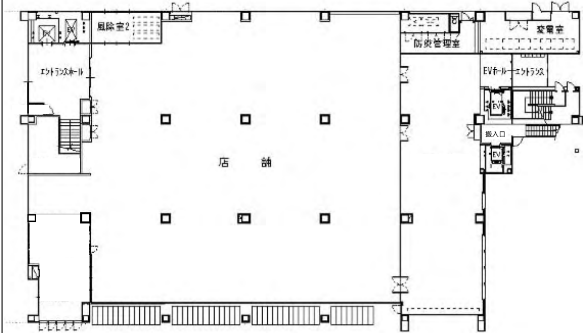
1階平面図
