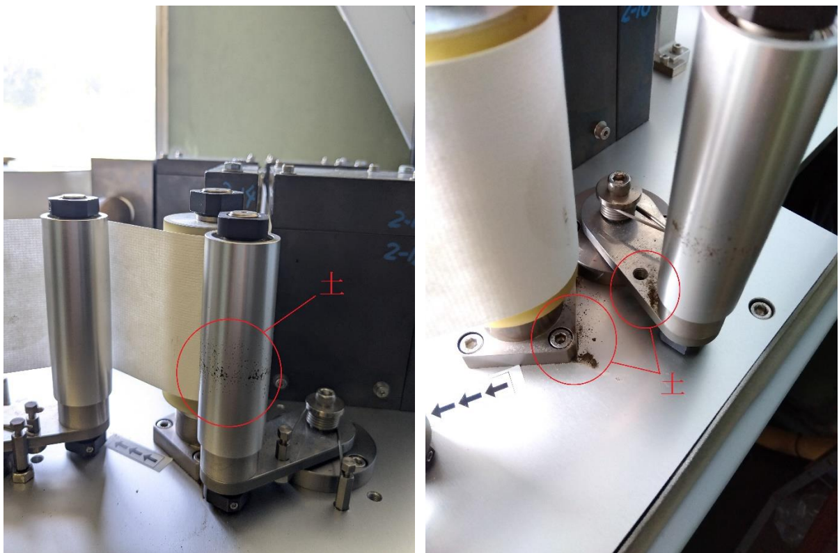
図2 ダストサンプラーろ紙送り部分
